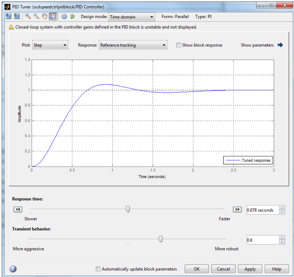
Displaying PID Parameters
